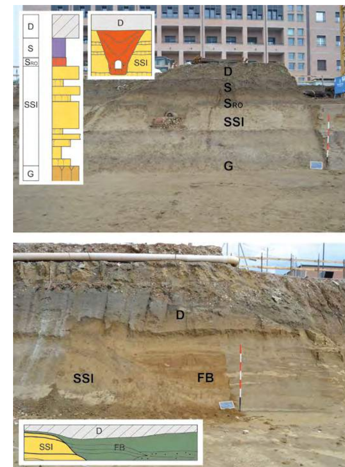
Fig. 1. Cantiere Ospedale, il paleoalveo protostorico del Crostolo e la fossa dell'acquedotto di età romana. D: riporti recenti; S: suolo attuale; Sro: suolo d'età romana; SSI: sabbie e limi; FB: sedimenti del paleoalveo del Crostolo; G: ghiaie.
