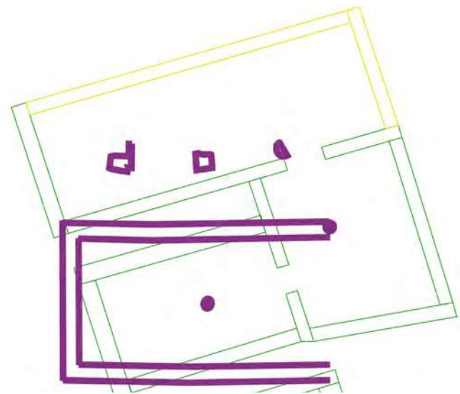
Fig. 5. Piazza della Vittoria, planimetria schematica dell'edificio 1, sovrapposta alla pianta della domus di età imperiale.
