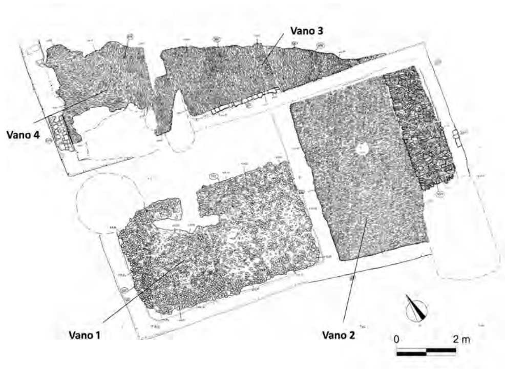
Fig. 6. Pianta del sottofondo dei pavimenti della domus : la linea divisoria a N (fra i vani 3 e 4) e la variazione di tecnica esecutiva a S/E alludono a fasi edilizie differenti.
