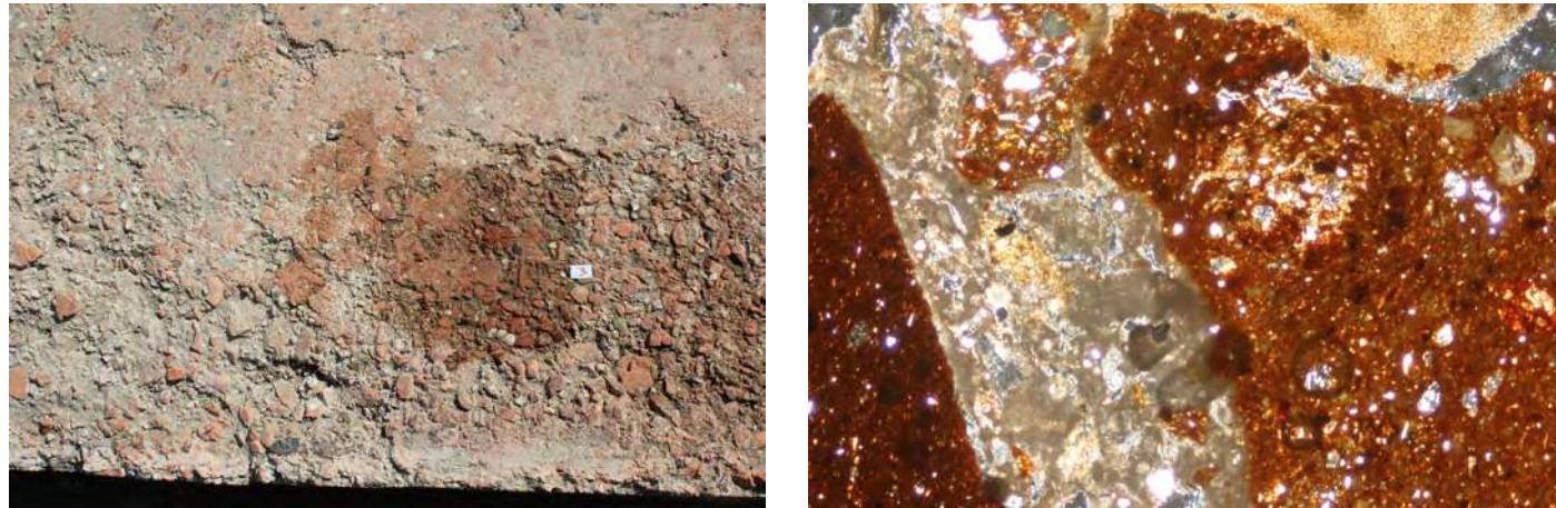
Fig. 3. A sinistra: ripresa della superficie dell'US 385. A destra la ripresa al microscopio dello strato interno: impasto rossiccio confezionato mescolando calce aerea, frammenti macinati di laterizi e granuli carbonatici. Sezione sottile 20 X.
